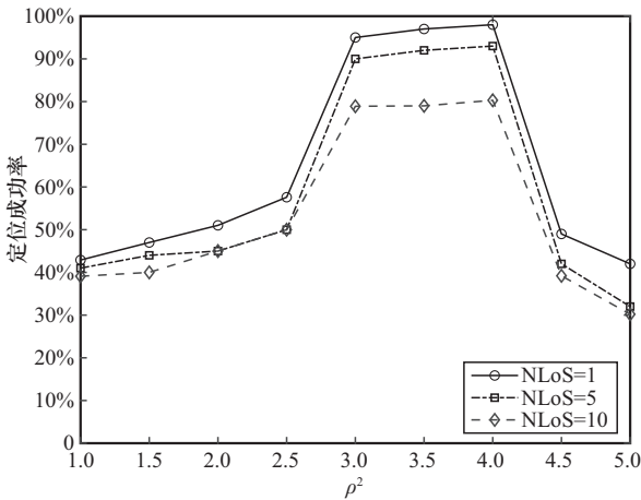
图3 不同 NLoS 路径数下 RDC 的定位成功率随参数 \rho^2 的变化特性
